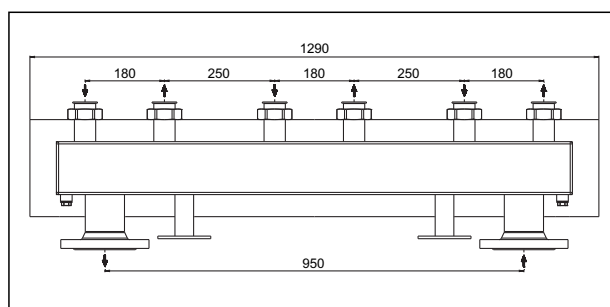
Распределительная гребенка Ду40/50 на 3 отвода
