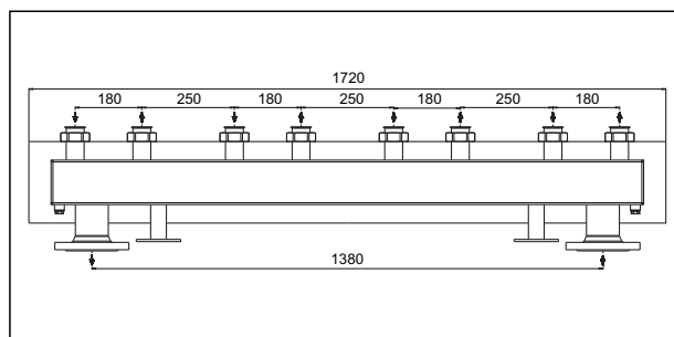
Распределительная гребенка Ду40/50 на 4 отвода
