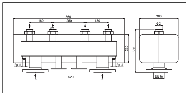
Распределительная гребенка Ду40/50 на 2 отвода
